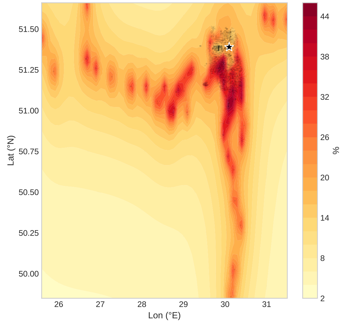
Eu154 (Mean 12.0 %)
