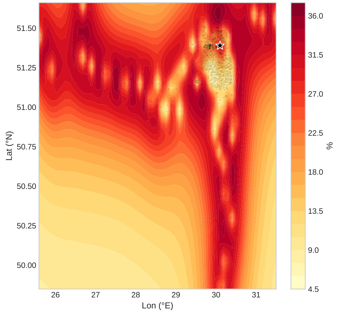
Sr90 (Mean 21.7 %)
