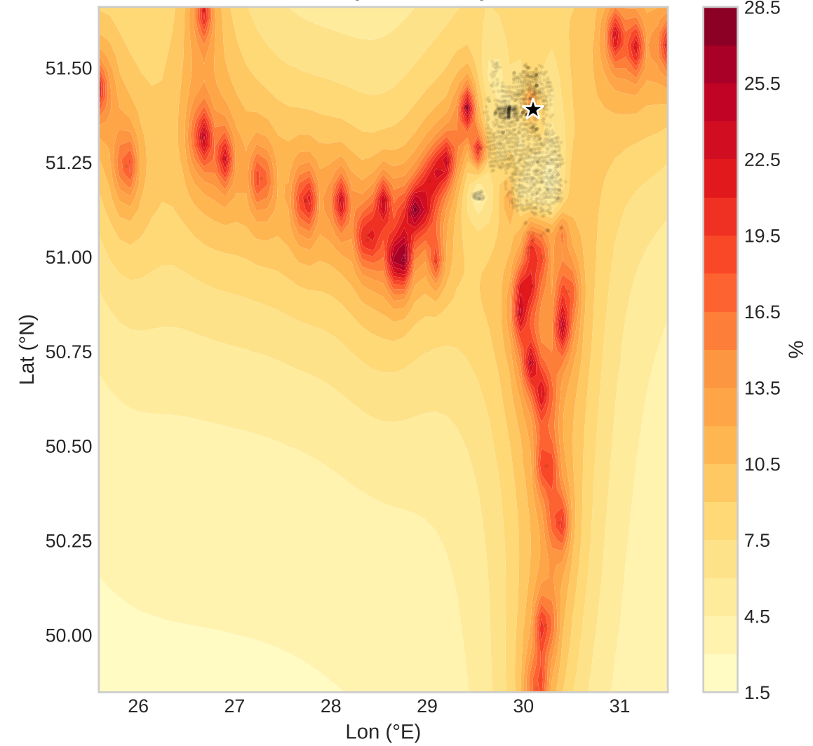
Pu238 (Mean 23.2 %)
